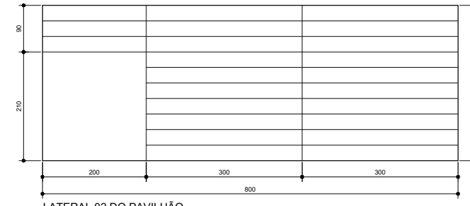
LATERAL 02 DO PAVILÃO
