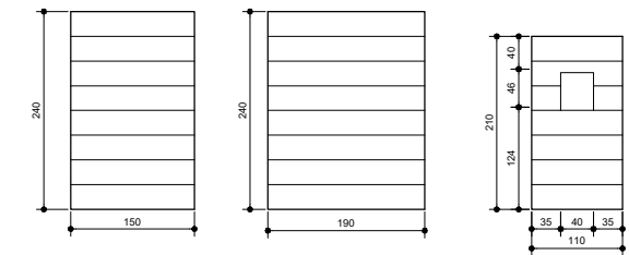
DETALHES VARANDA
