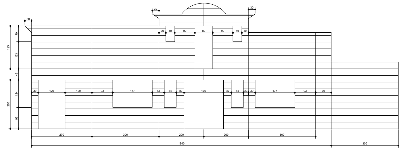
FACHADA DO PAVILÃO - MEDIDAS
