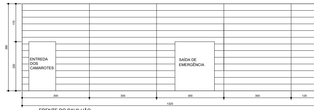
FRENTE DO PAVILÃO
