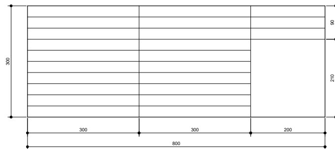
LATERAL 01 DO PAVILÃO
